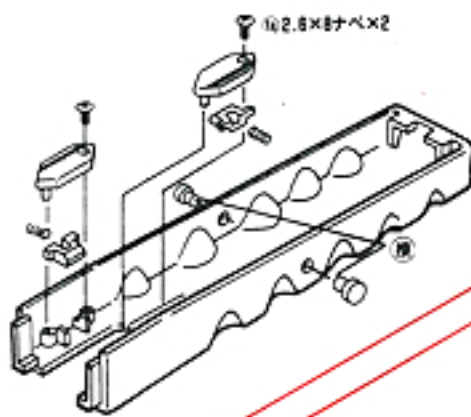
FH-8 5.56F1 フォアグリップ
