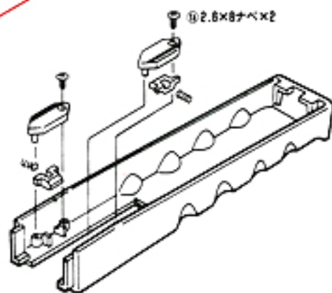
SV-8 SUPER VERSION フォアグリップ
